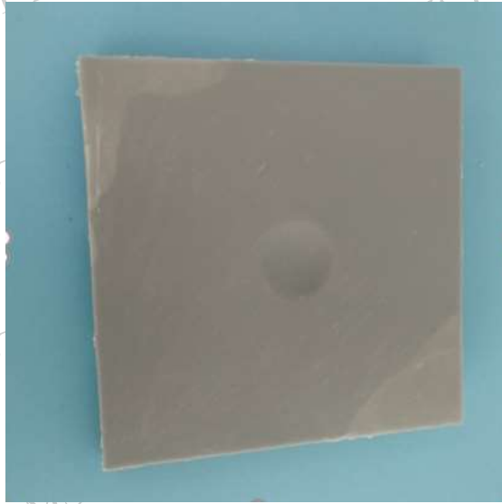
图 6-30%亚硫酸试验后照片 Photo 6-after 30% sulfite test
