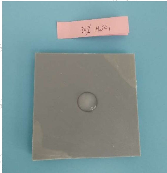
图 5-30%亚硫酸试验中照片 Photo 5-in 30% sulfite test
