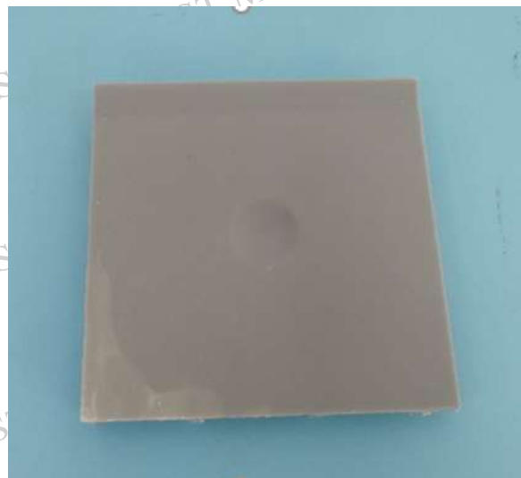
图 9-30%硝酸试验后照片 Photo 9-after 30% nitric acid test
