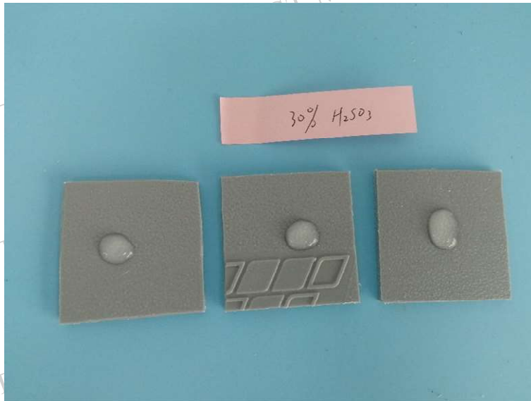
图 5-30%亚硫酸试验中照片 Photo 5-in 30% sulfite test
