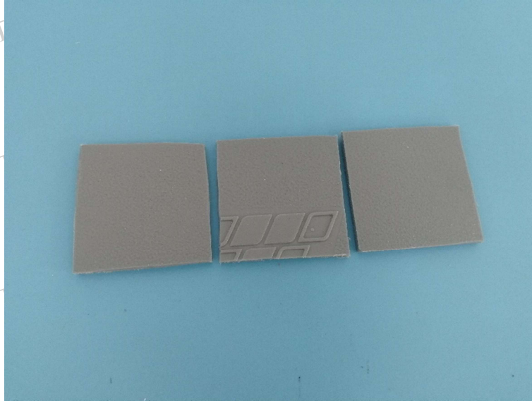
图 6-30%亚硫酸试验后照片 Photo 6-after 30% sulfite test
