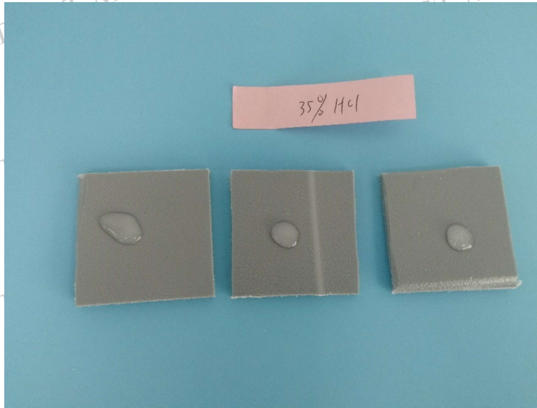
图 2-35%盐酸试验中照片 Photo 2-in 35% hydrochloric acid test
