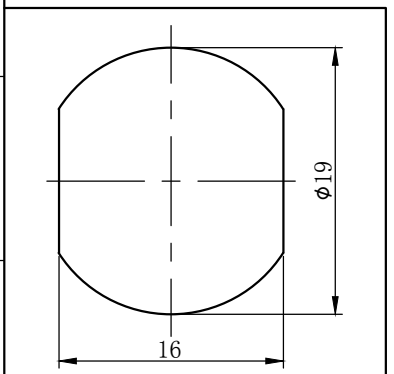
パネル穴明け寸法
