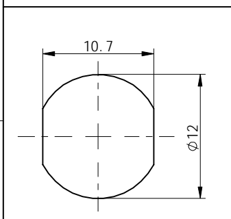
取付穴図
